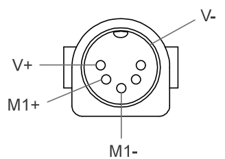
Prise DIN Type U 5 broches
