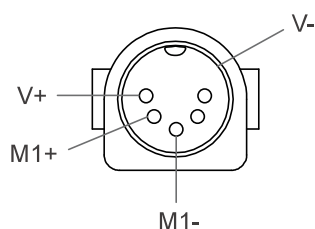
Prise DIN Type U male 5 broches
