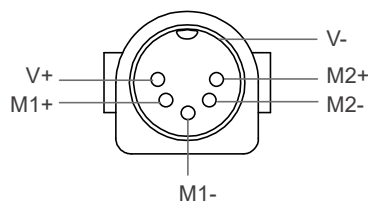
Brochage du connecteur : C-DIN-52R
