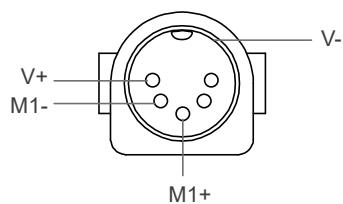
Brochage du connecteur : C-DIN-51H
