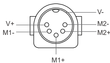
Brochage du connecteur : C-DIN-52H
