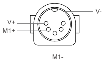
Brochage du connecteur : C-DIN-51R
