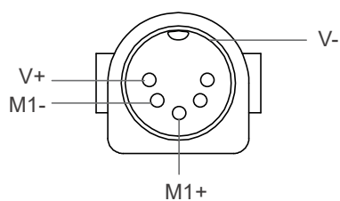
Prise DIN Type U 5 broches Male (Brochage du connecteur : C-DIN-51H)
