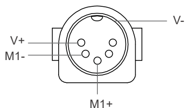
Prise DIN Type U 5 broches Male (Brochage du connecteur : C-DIN-51H)
